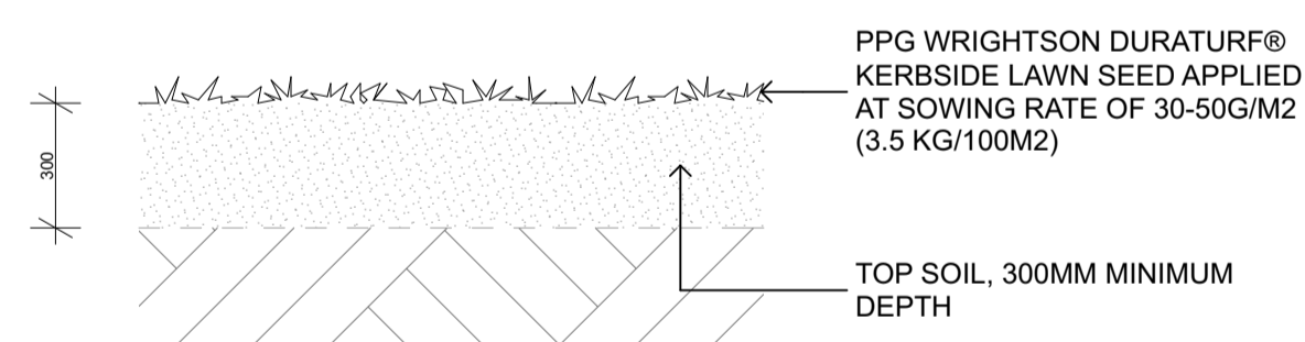
PD-06: LAWN 1:20@A1 / 1:40@A3
