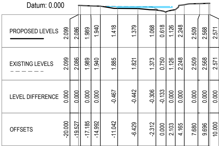
CHAINAGE 40.000
