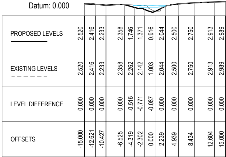
CHAINAGE 100.000
