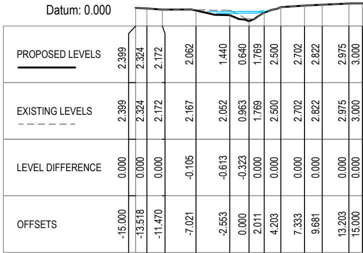
CHAINAGE 80.000
