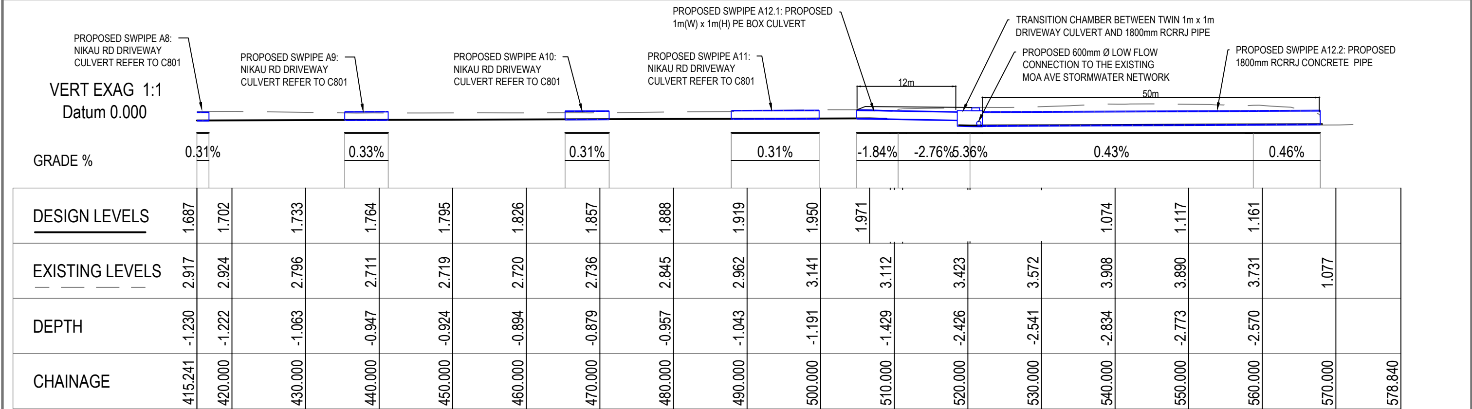
TUI-NIKAU LONG SECTION
