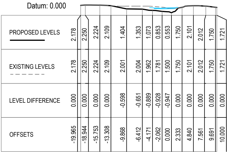
CHAINAGE 00.000
