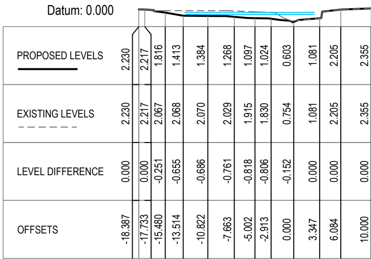
CHAINAGE 20.000
