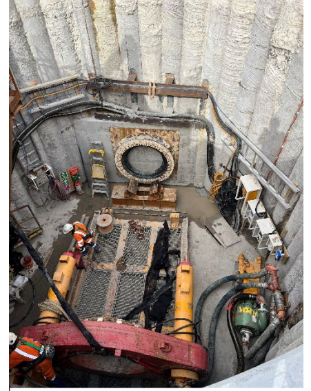
TBM प्रवेश द्वार - एम्ब्रिको प्लेस दस्ता
