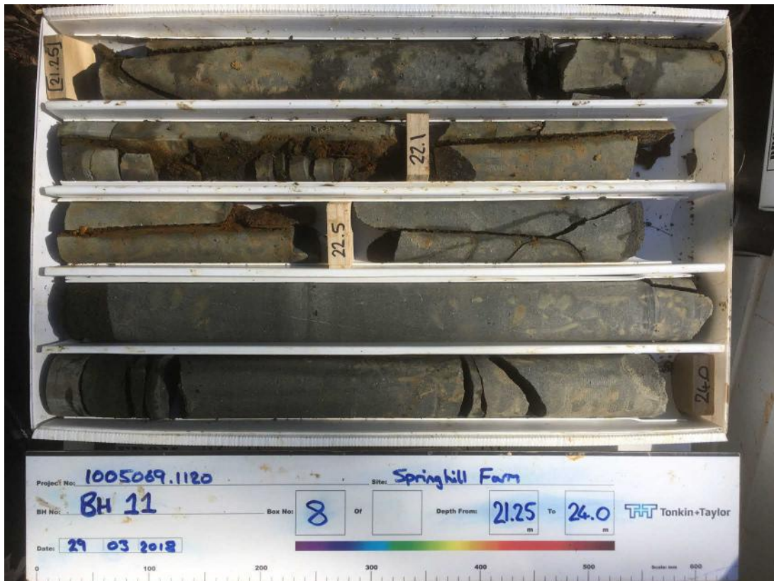
BH11_Core Box 8 (1)
