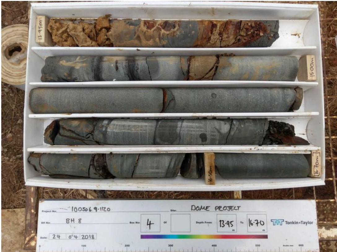
BOX 4 13.95-16.70m
