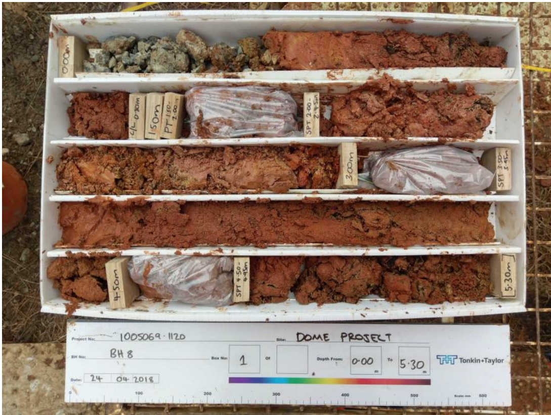
BOX 1 0.00-5.30m
