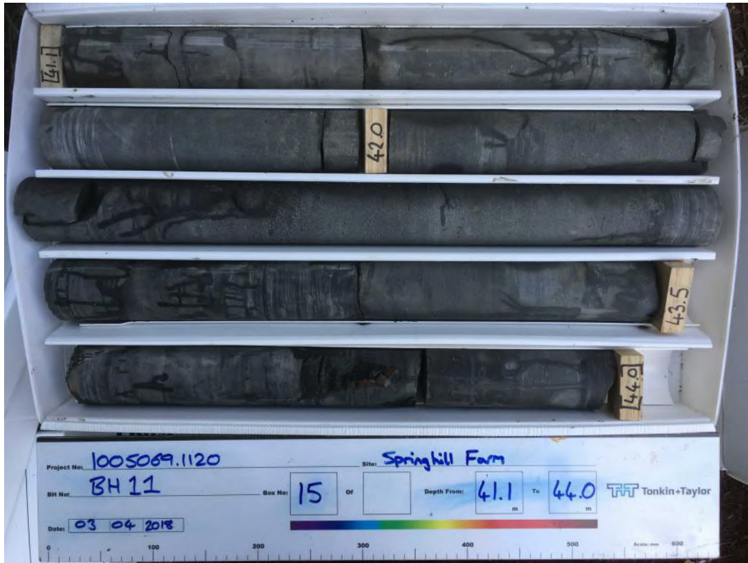
BH11_Core Box 15 (1)
