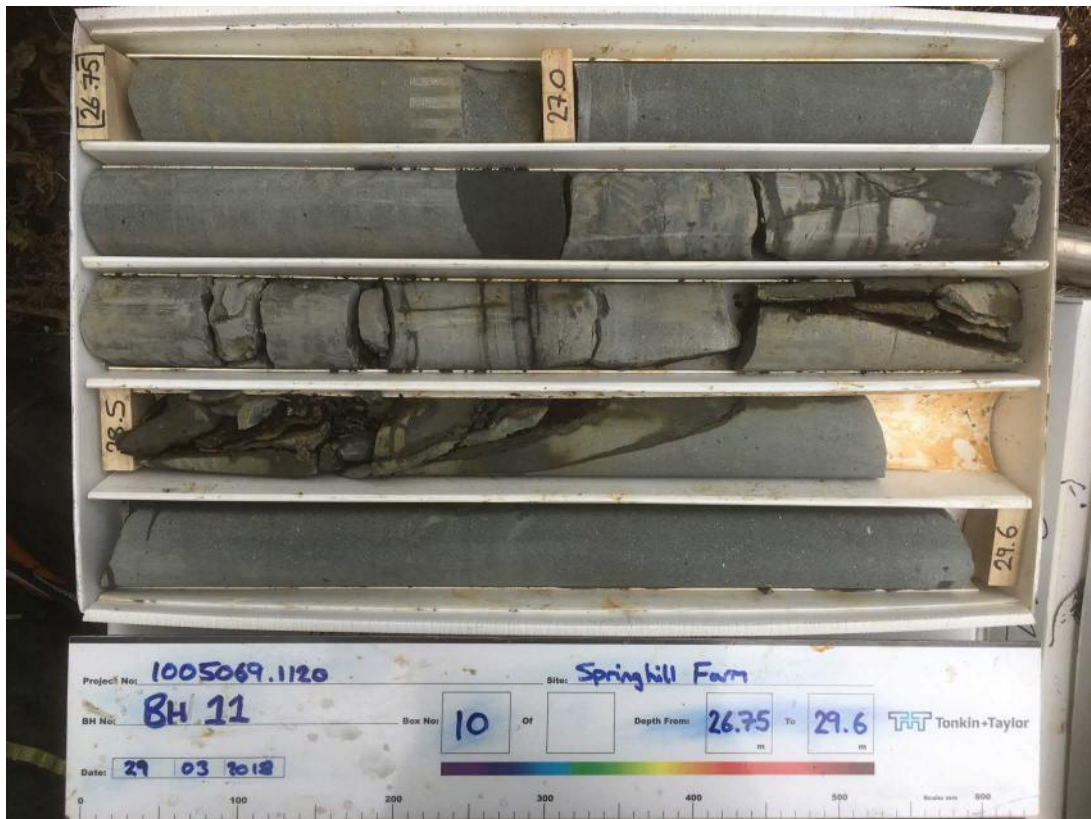
BH11_Core Box 10 (1)
