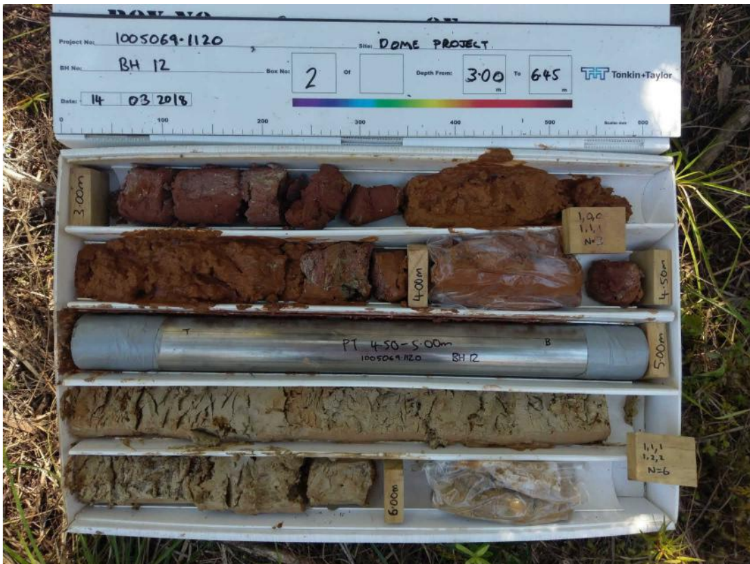
BOX 2 3.00-6.45m
