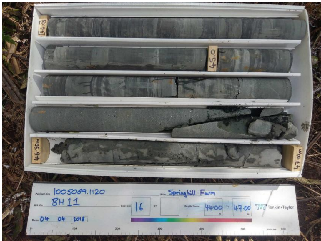
BH11_Core Box 16
