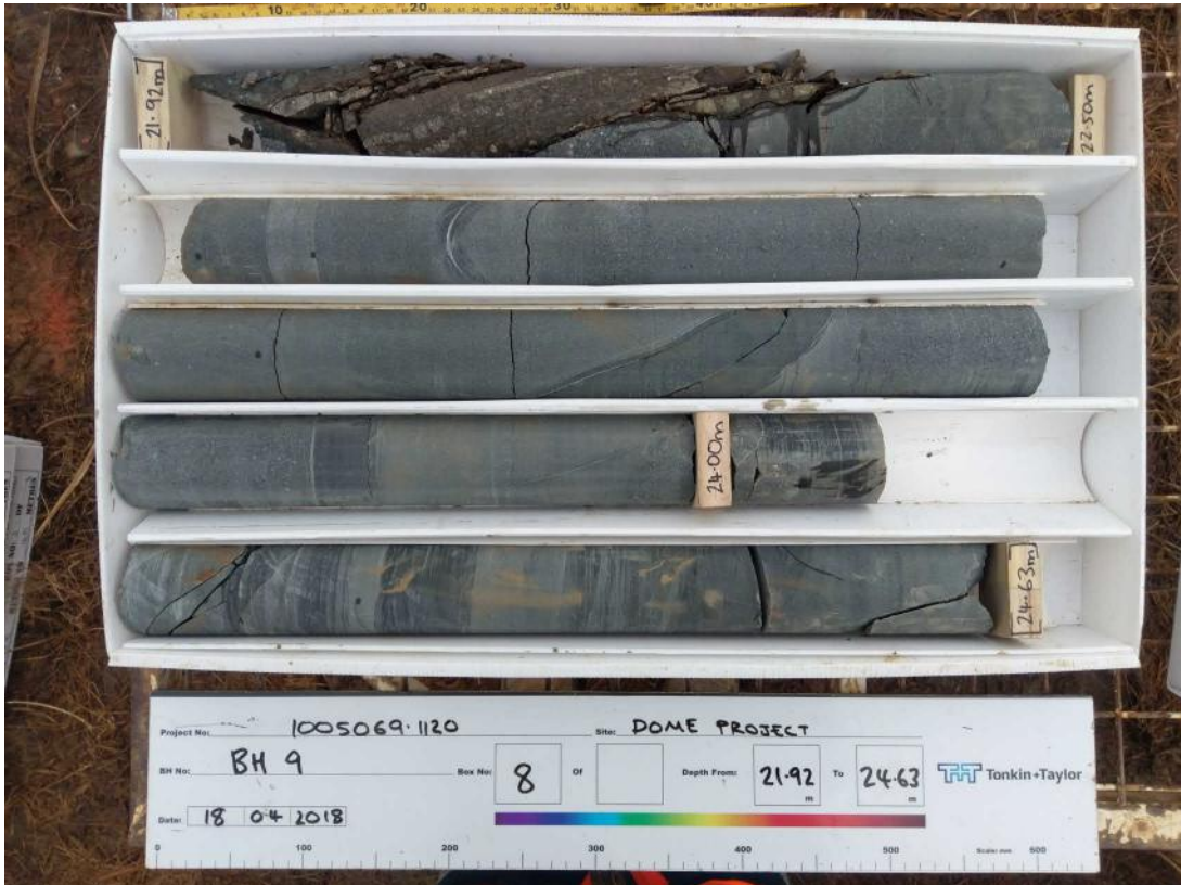
BOX 8 21.92-24.63m
