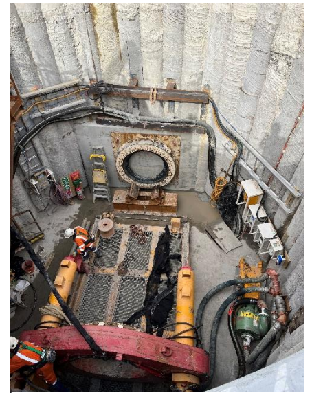
TBM入口——Ambrico Place竖井
